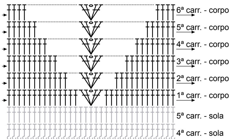
Diagrama - Corpo do sapato
