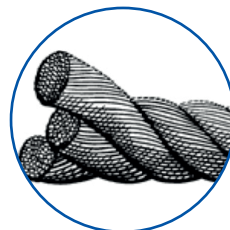
DETALHE DO FILAMENTO E CONSTRUÇÃO DA LINHA CORRENTE POLI MATÊ
